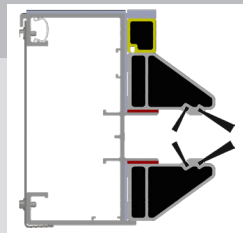
Espacio de perfil compacto con resistencias térmicas integrales
