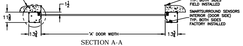
SECTION A-A
