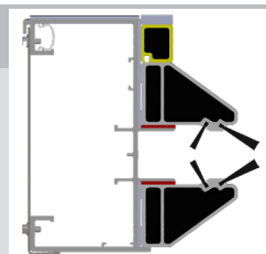
Empreinte bas profil avec barrières thermiques intégrées
