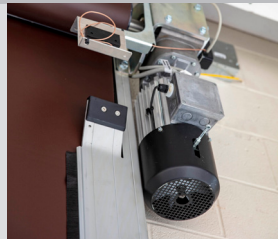
Motor con transmisión directa
